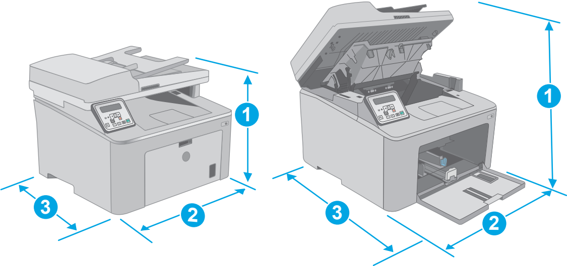
图 1-1 打印机尺寸
