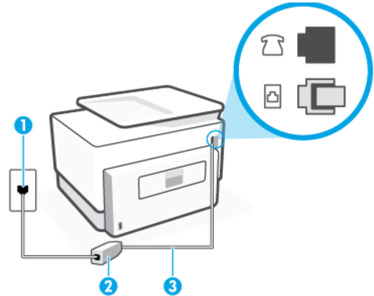
图 4-2 打印机的后视图
