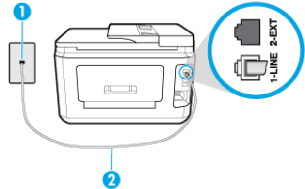
图 5-5 打印机的后视图
