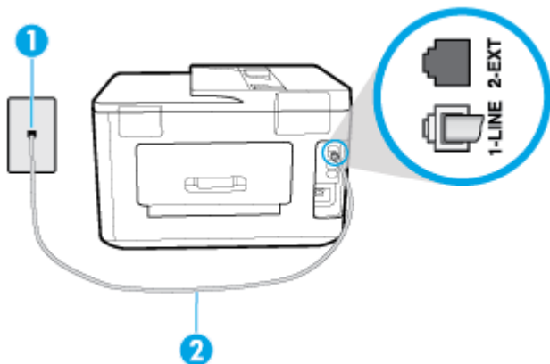
图 5-3 打印机的后视图
