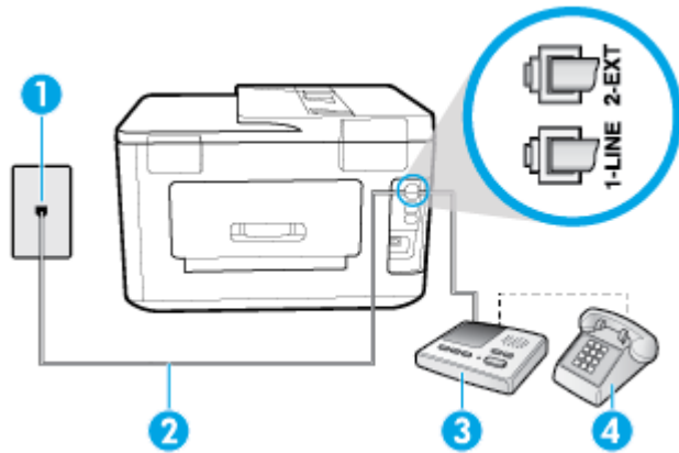
图 5-11 打印机的后视图
